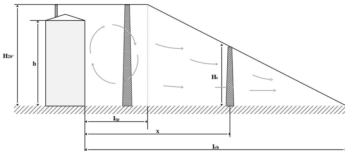
Figure 3: Détermination de la hauteur de la cheminée en considérant des bâtiments hauts isolés.
